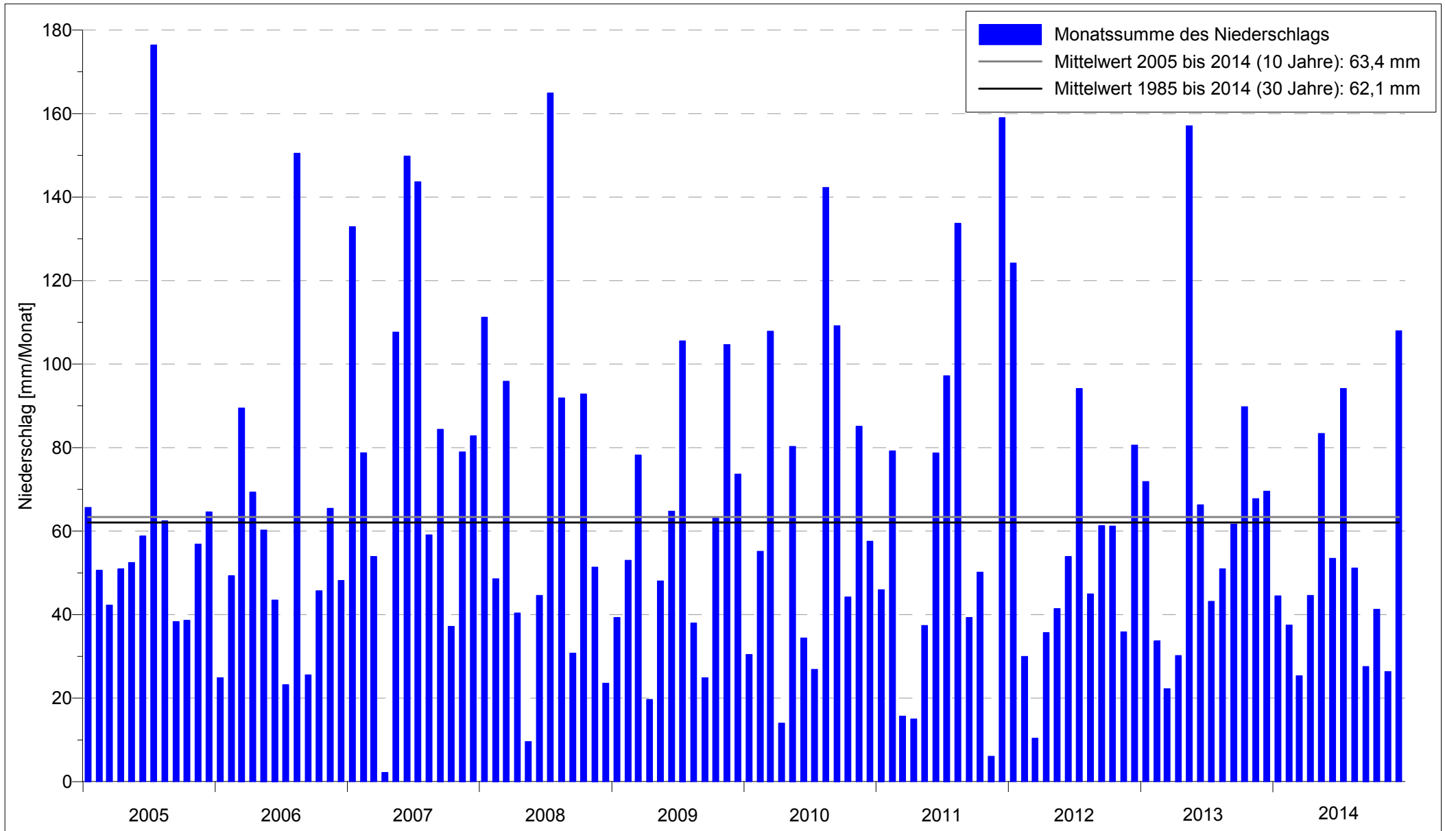
Anl. 4: Monatssummen der Niederschläge, DWD-Station Neuwiedenthal, Zeitraum 01.01.2005 - 31.12.2014
