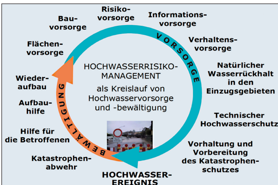
Abbildung 2: Der Hochwasserrisikomanagementkreislauf [2]
