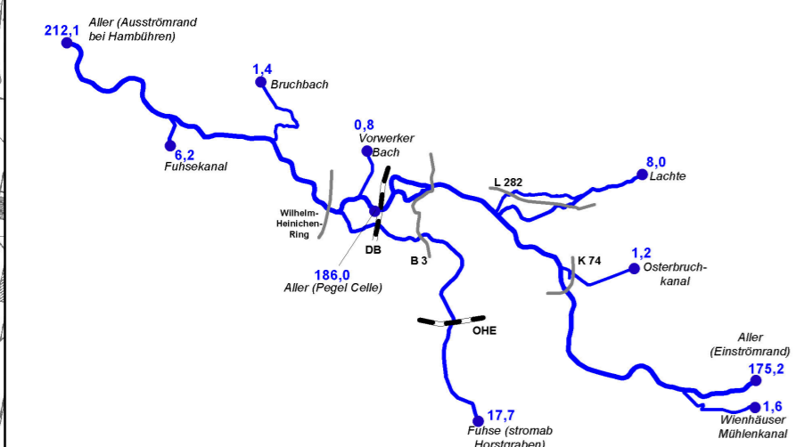
Abflussaufteilung für das Szenario HQ10 am Pegel Celle
