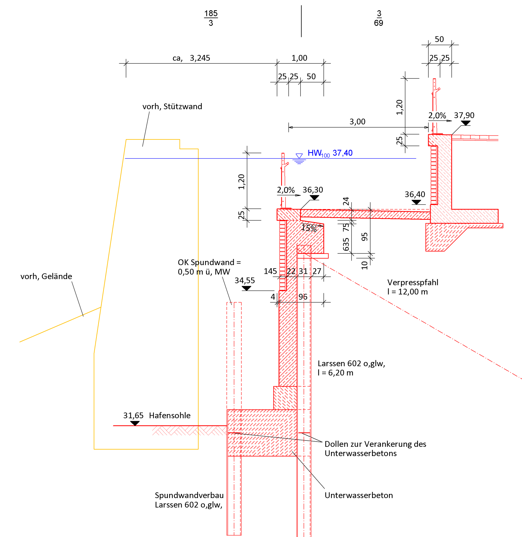
Schnitt O-O Hafenmauer Nord
