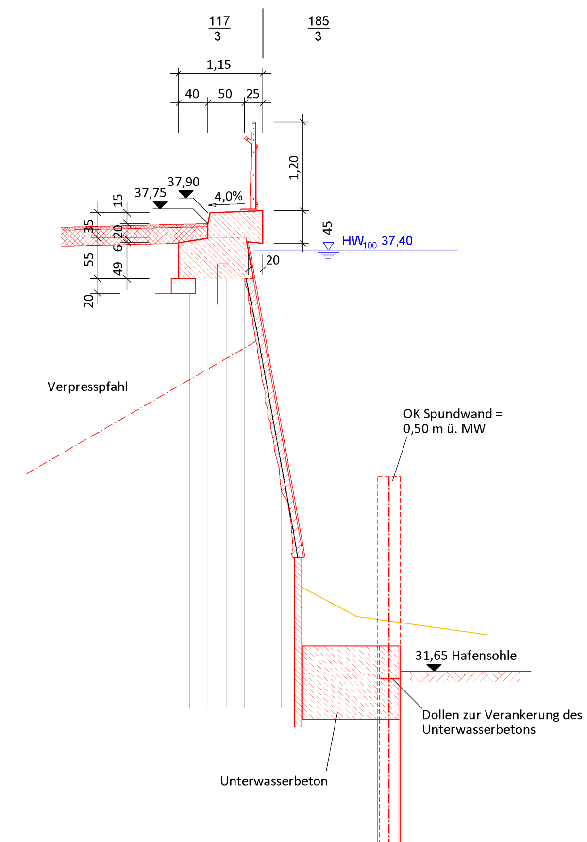
Schnitt Q-Q Hafenmauer Süd
