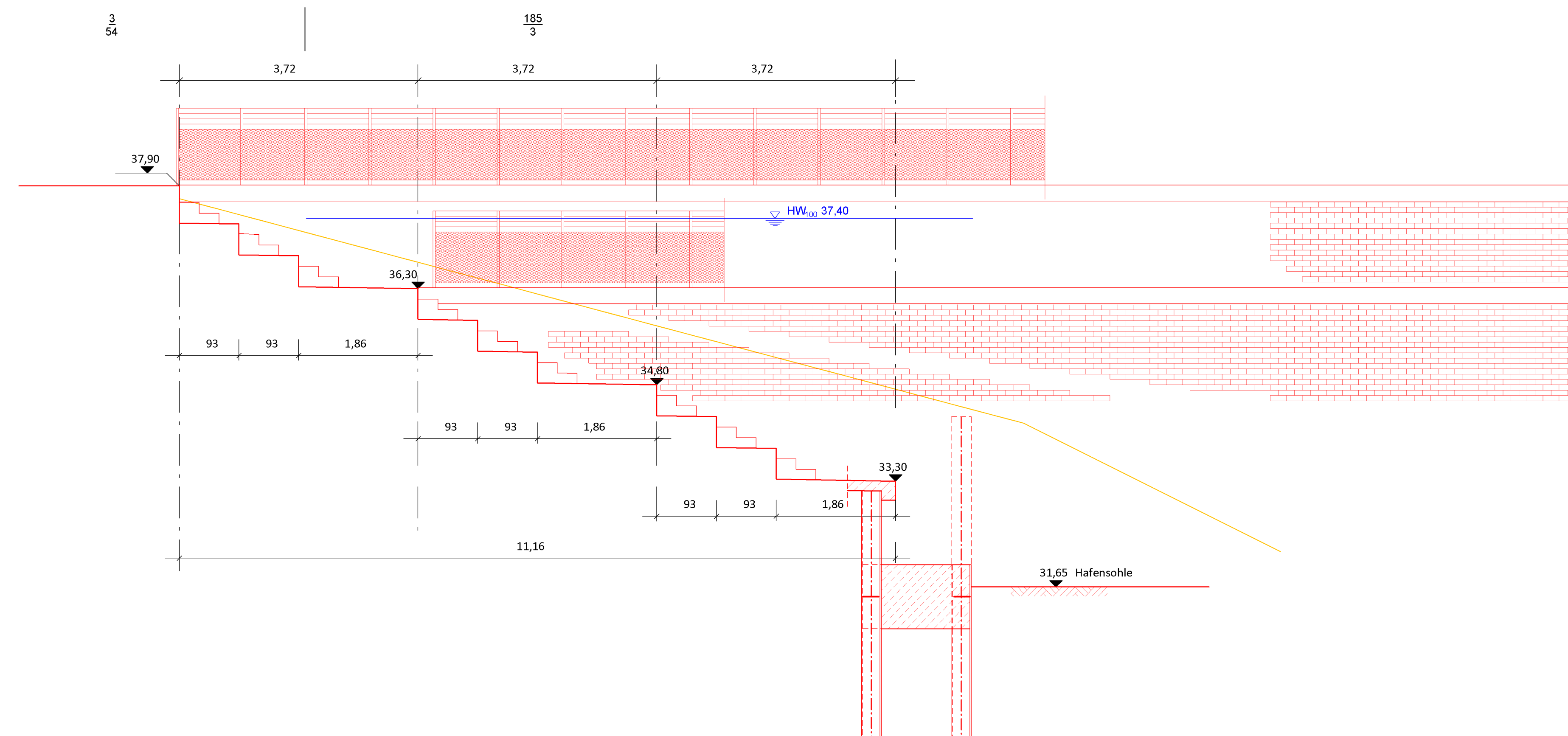
Schnitt P-P Rampenanlage West
