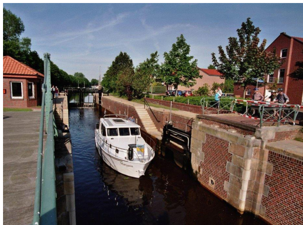
Emsschleuse Haren-Rütenbrock-Kanal
