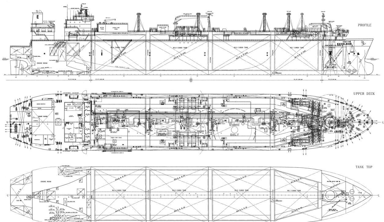
Abbildung 2-5: Allgemeiner Übersichtsplan der Excelsior
