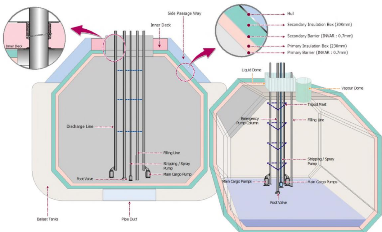
Abbildung 2-23: LNG-Tanks der Excelsior
