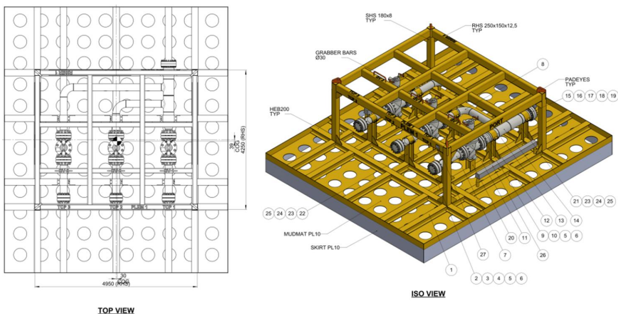
Abbildung 2-15: PLEM am Meeresboden
