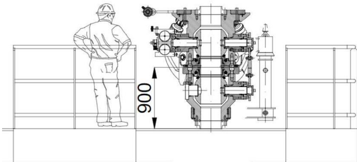
Abbildung 2-11: ERS-Notentriegelungssystem
