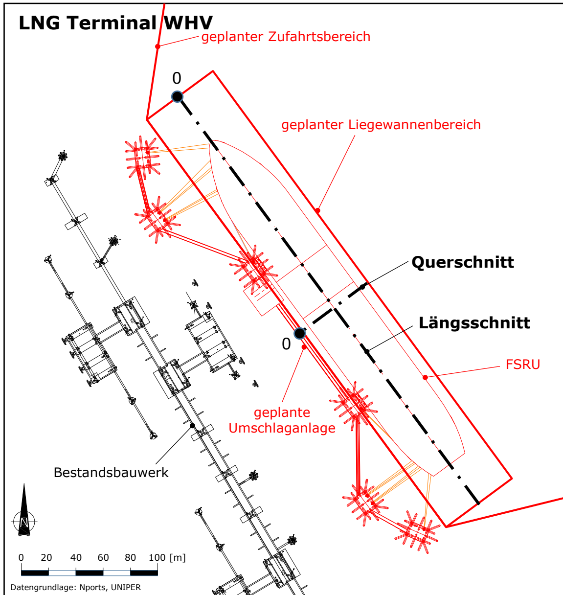
Lage der Schnitte (Prinzipsskizze)
