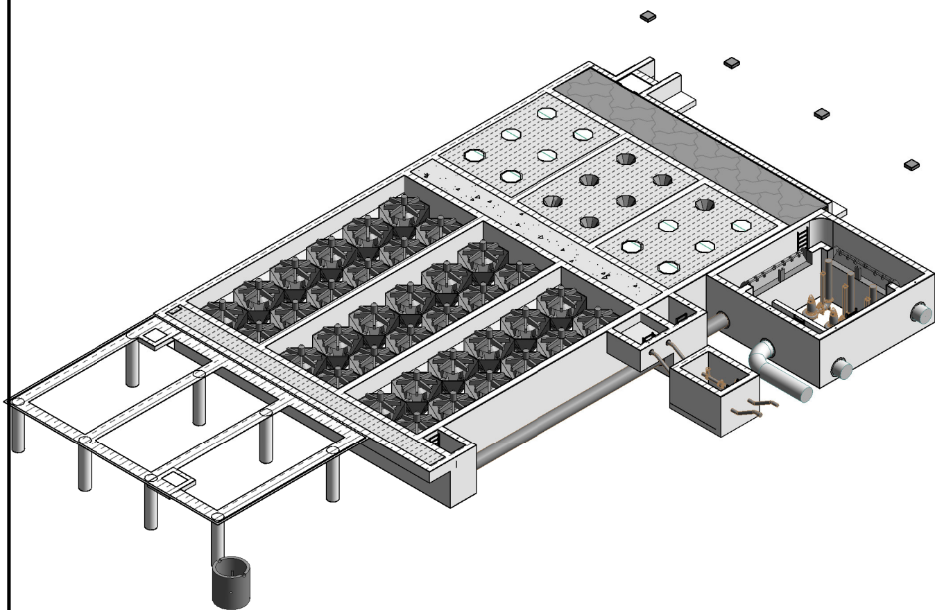
3D-Übersicht auf +89.20 NHN
