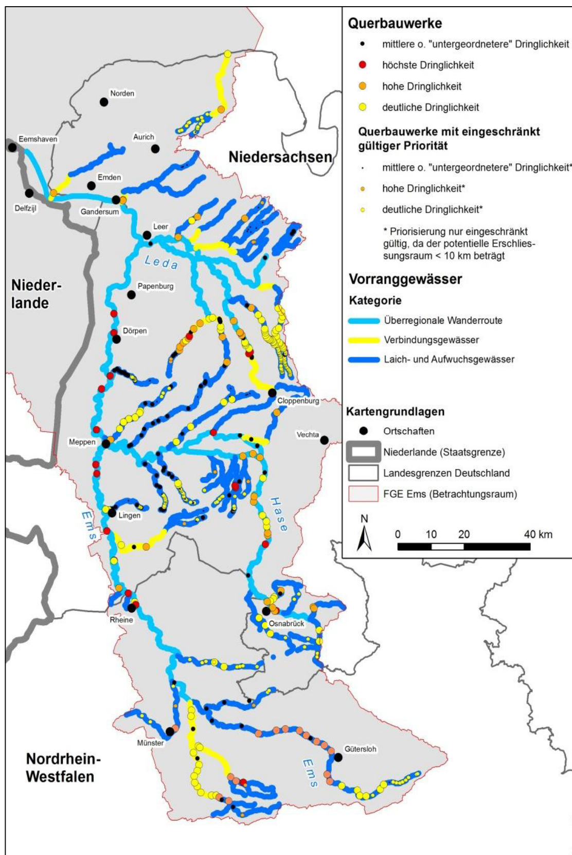
Abb. 5-6: Vorranggewässer für die Herstellung der Durchgängigkeit - Einstufung der Maßnahmendringlichkeit (FGG EMS 2012) aus FGG EMS (2020b)
