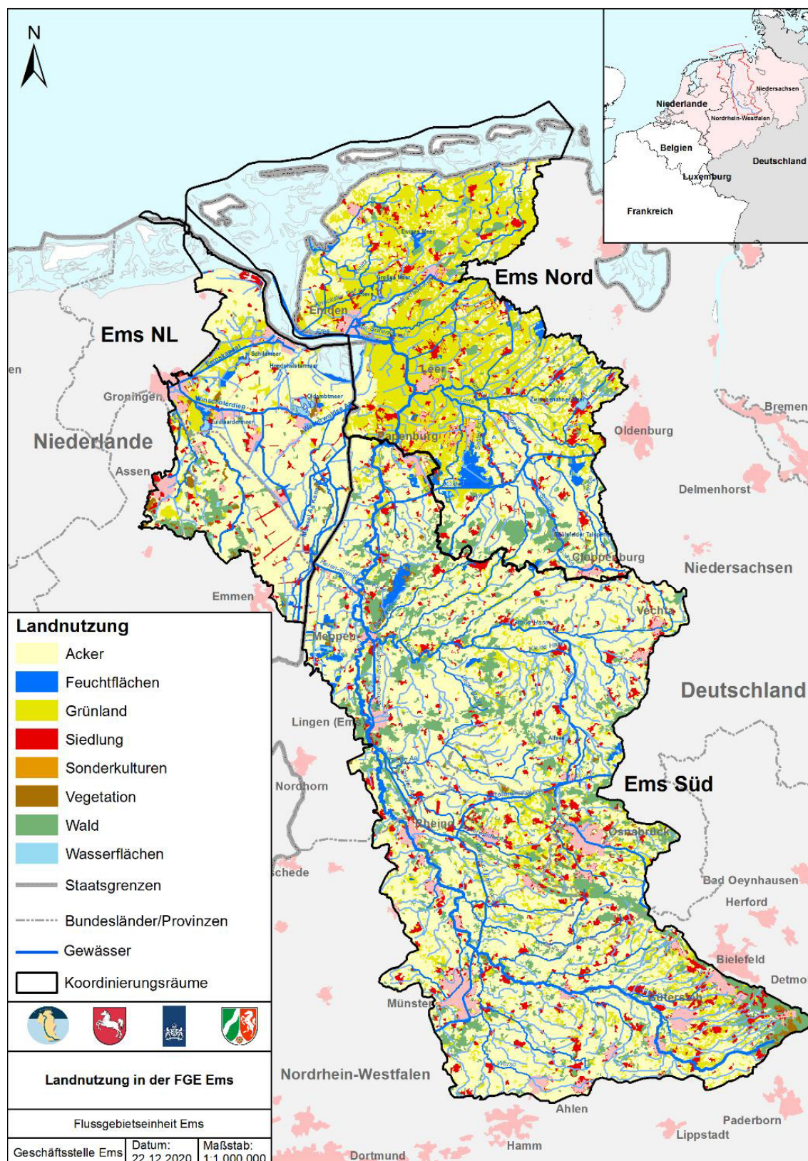
Abb. 5-8: Landnutzung und Bodenbedeckung in der FGE Ems (ohne Küstengewässer, CO-RINE LANDCOVER 2018 (European Environment Agency 2020)) aus FGG EMS (2020a)
