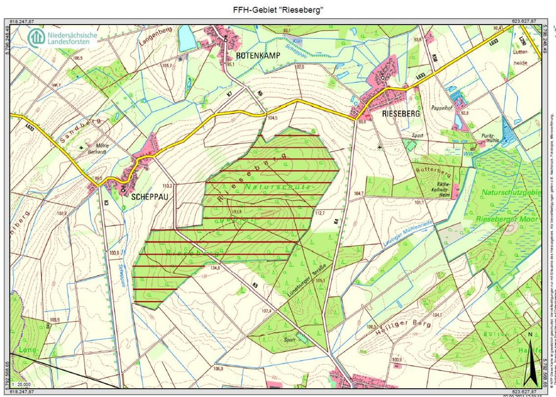
Abb.: Übersichtskarte FFH-Gebiet „Rieseberg“.
