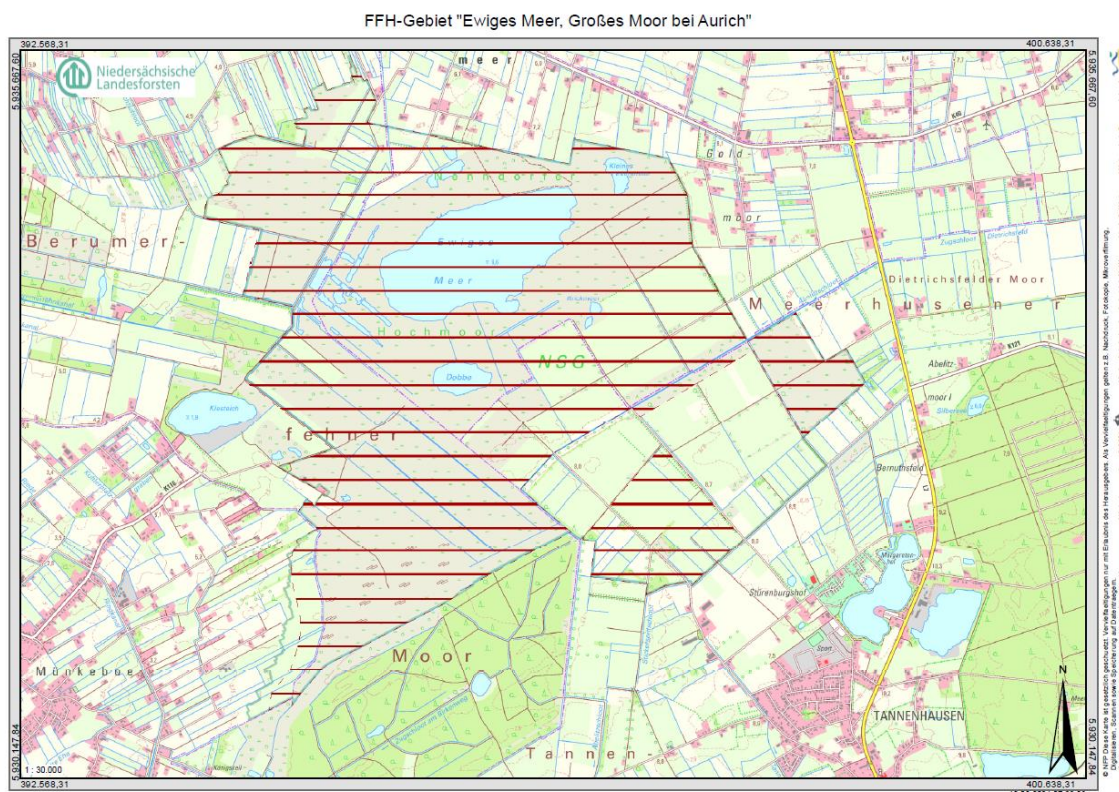
Abb.: Übersichtskarte FFH-Gebiet „Ewiges Meer, Großes Moor bei Aurich“
