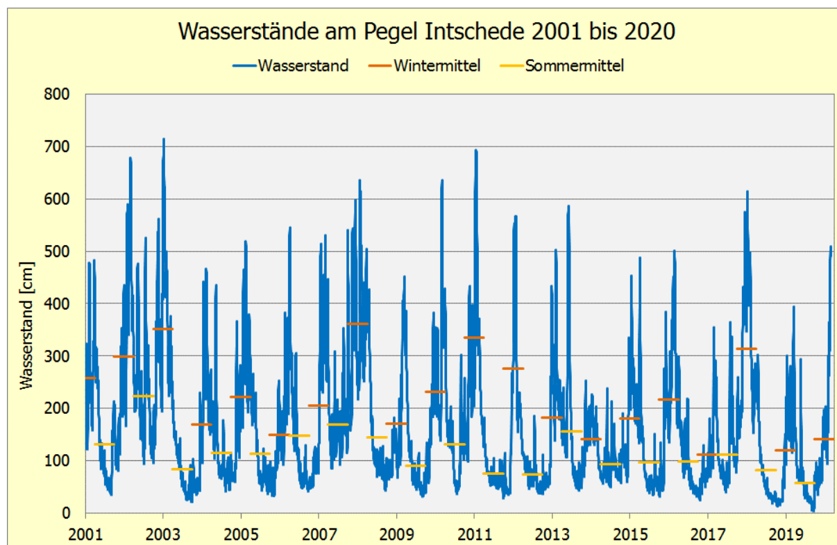
Abb. 2.3: Wasserstände am Pegel Intschede (Mittelweser, oberhalb von Bremen) (2001 bis 2020)
