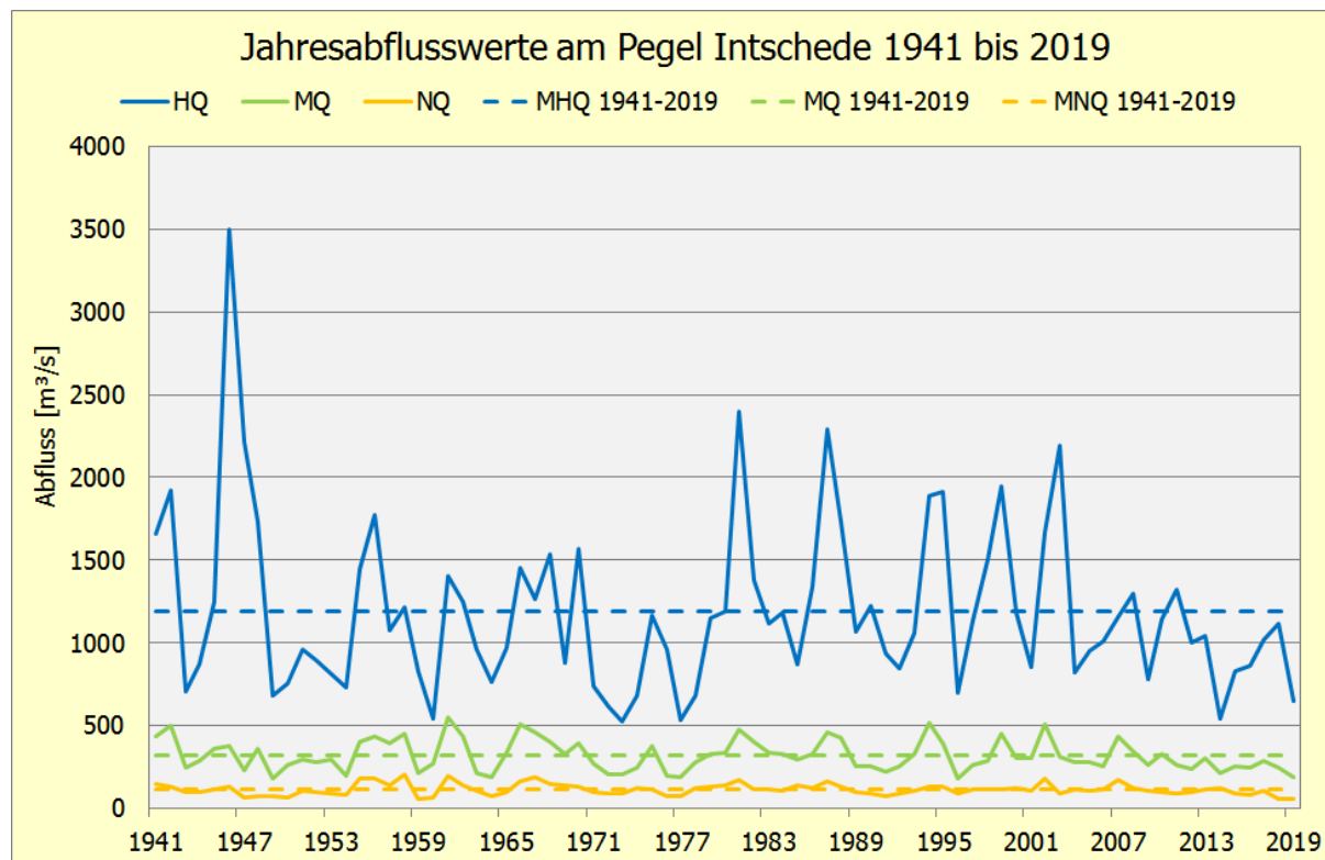
Abb. 2.4: Niedrigste, mittlere und höchste Jahresabflusswerte am Pegel Intschede 1941 bis 2019
