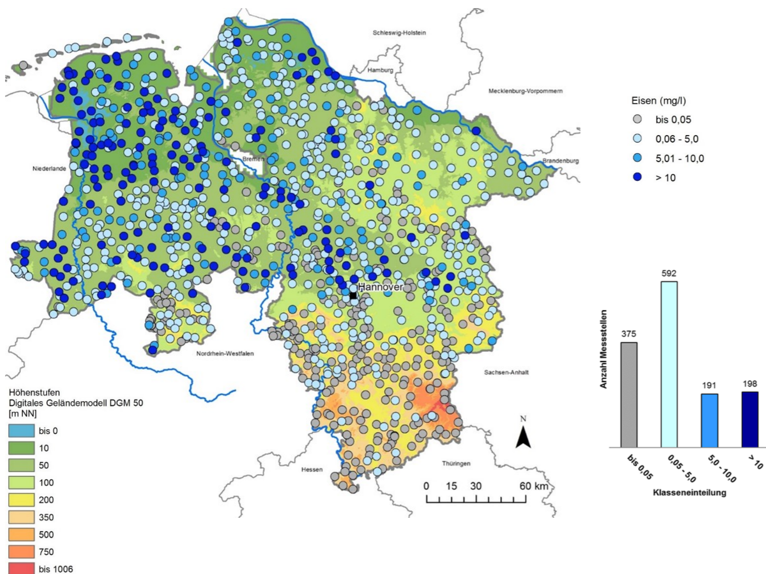
Abbildung 1: Eisengehalte im Grundwasser (Datenbestand 2018).
